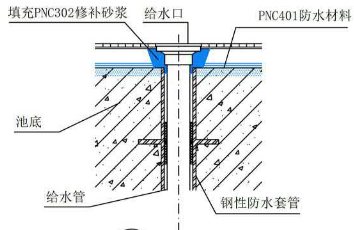
③ 池底给水口详图
