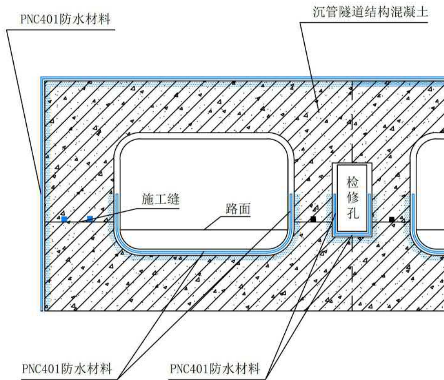
① 沉管隧道防水构造示意
