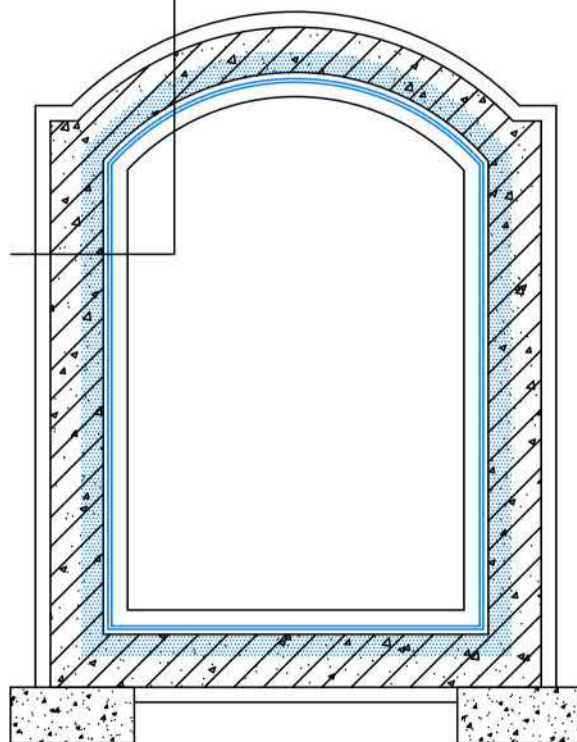
① 贴壁式洞库防水构造示意
