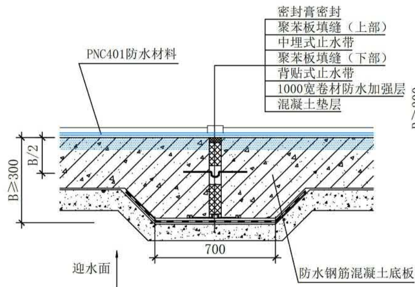
① 底板变形缝防水构造（一）
