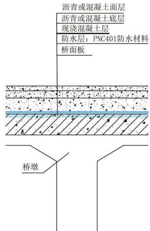
② 桥面板防水构造示意
