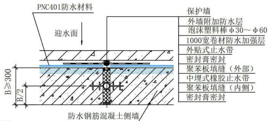
② 侧墙变形缝防水构造
