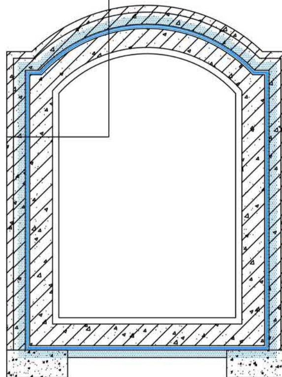
② 离壁式洞库防水构造示意
