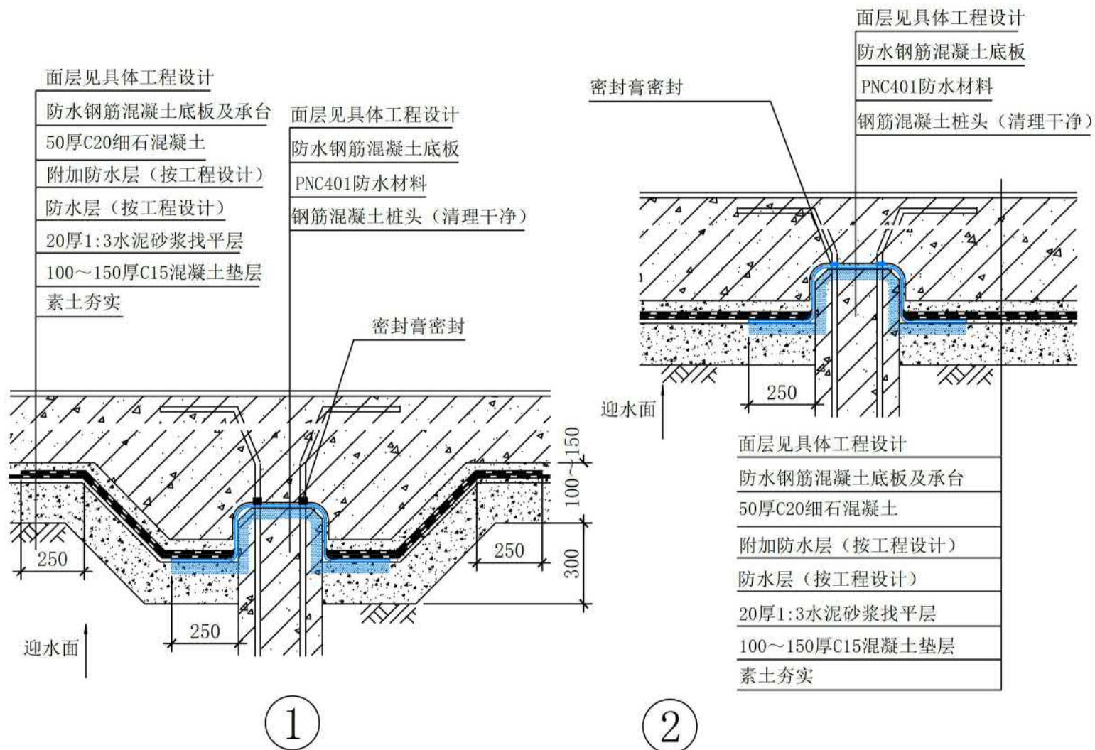
桩头防水构造-PNC401防水
