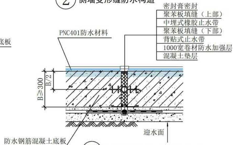
③ 底板变形缝防水构造（二）
