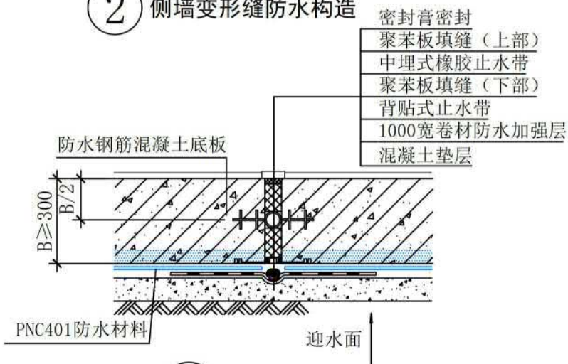
④ 底板变形缝防水构造 (二)
