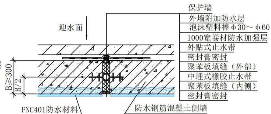
② 侧墙变形缝防水构造
