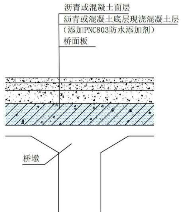
② 桥面板防水构造示意
