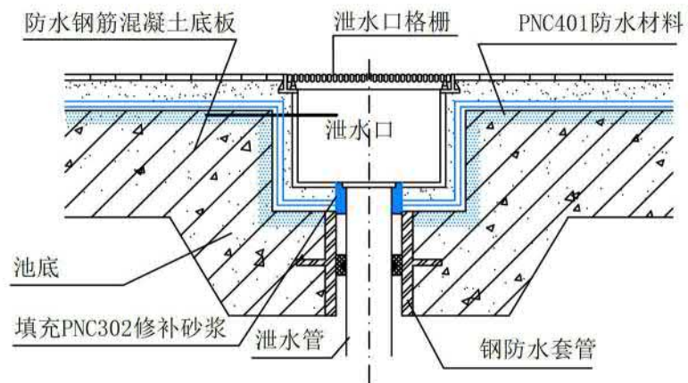
② 池底泄水口详图
