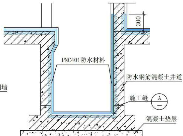
② 电梯井道防水构造
