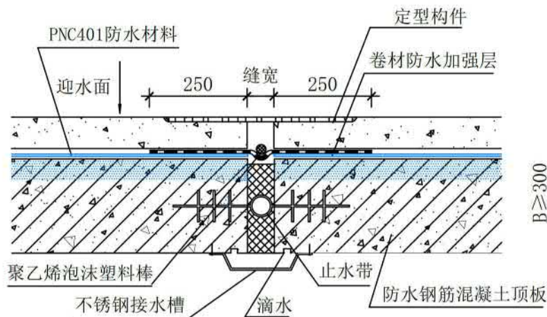
① 顶板变形缝
