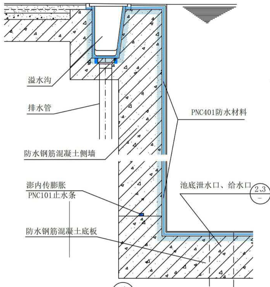
① 游泳池防水
